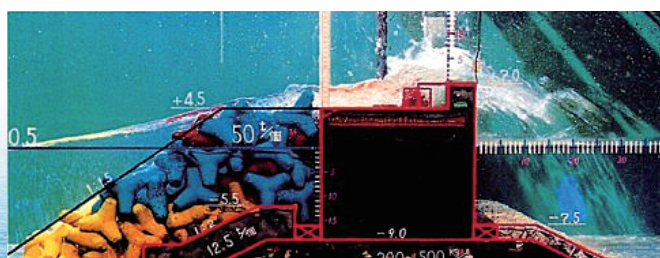
後部パラペット型防波堤断面実験
