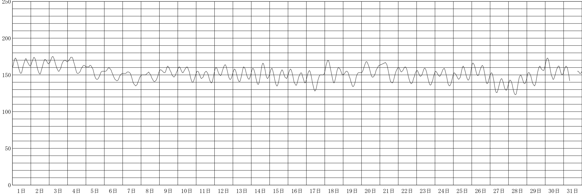
潮位 (cm) 2000年 10月
