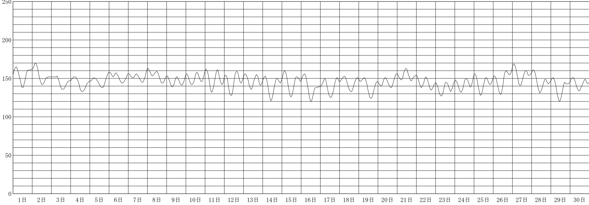
潮位 (cm) 2000年 11月
