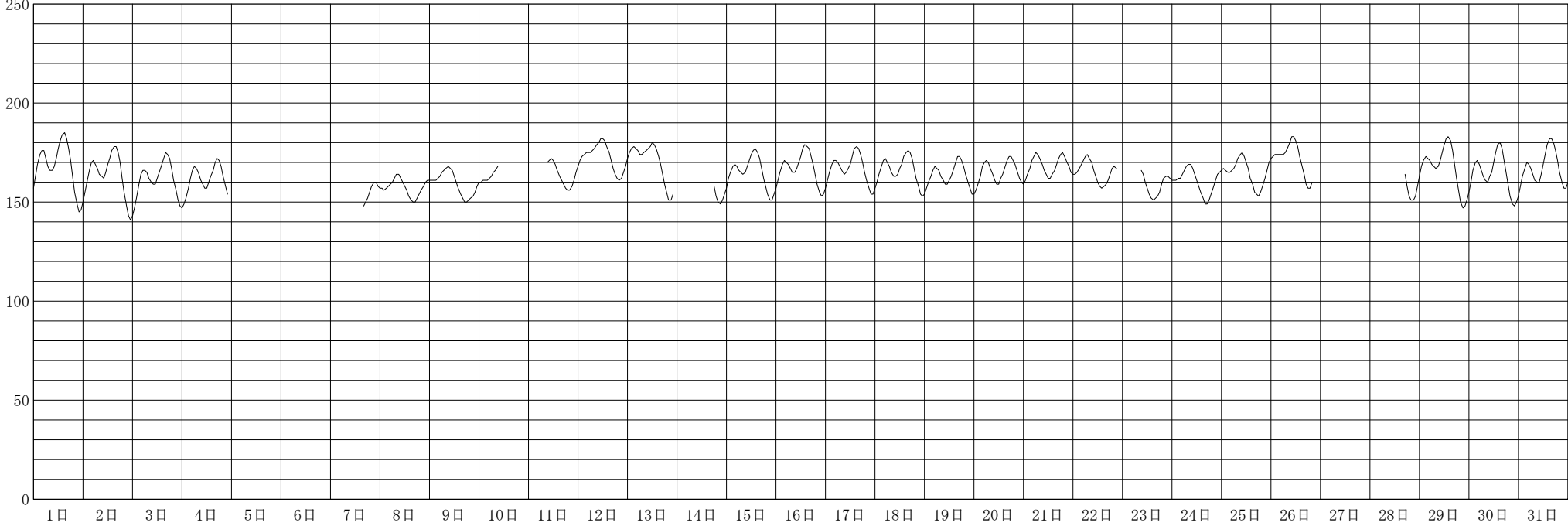
潮位 (cm) 2000年 8月
