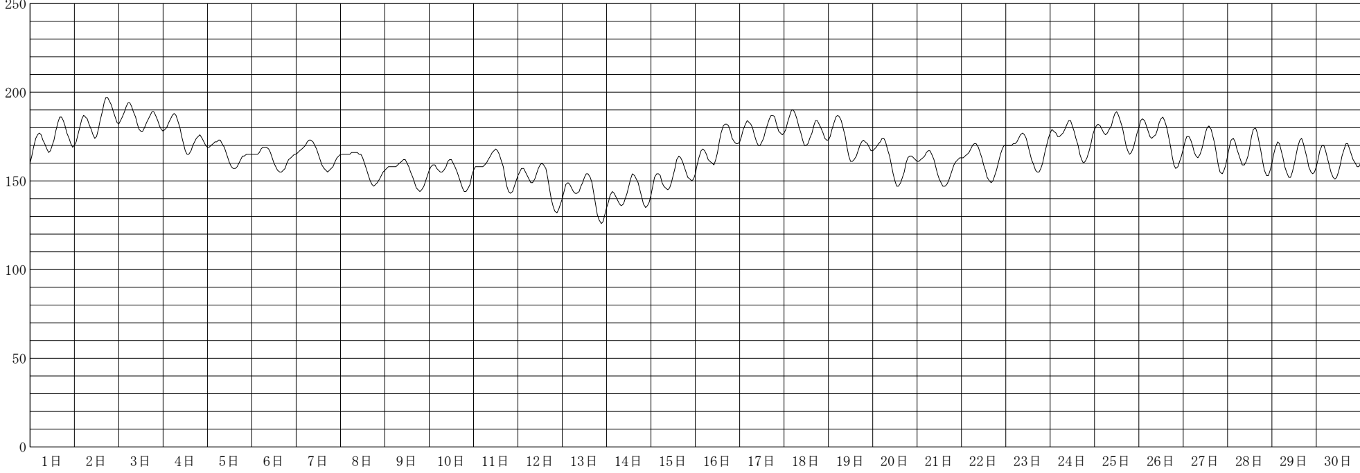
潮位 (cm) 2000年 9月
