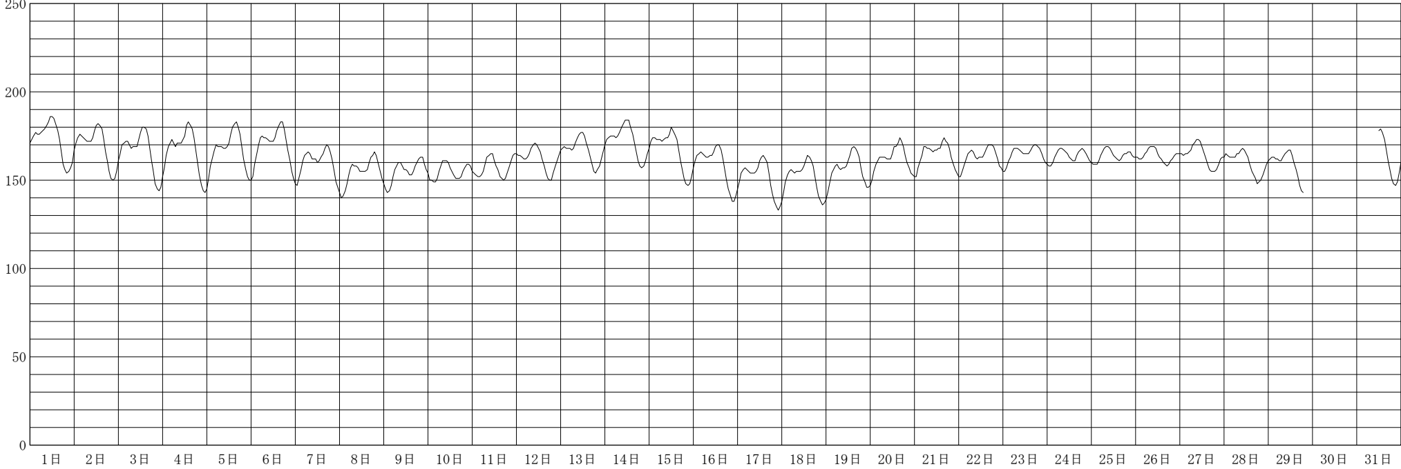
潮位 (cm) 2019年 7月
