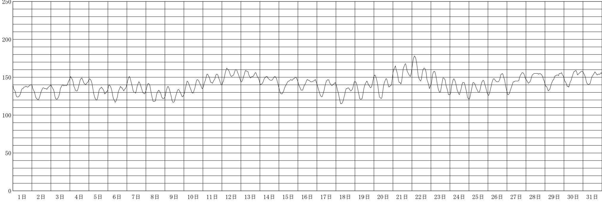
潮位 (cm) 2019年 3月
