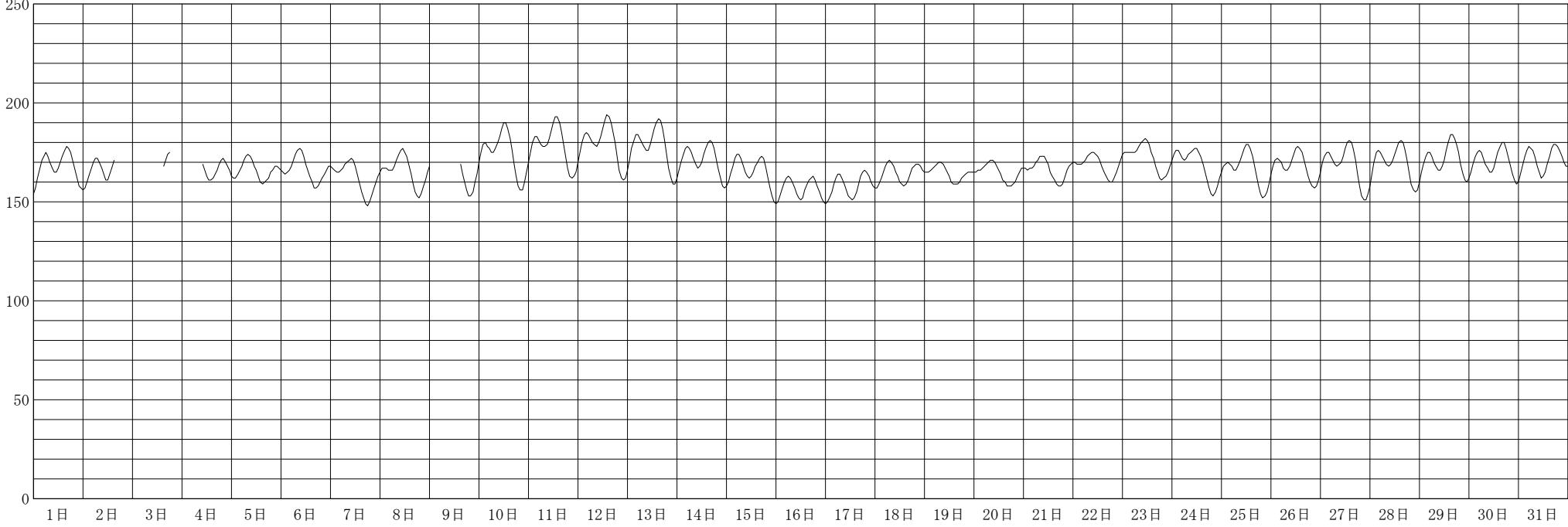
潮位 (cm) 1999年 8月
