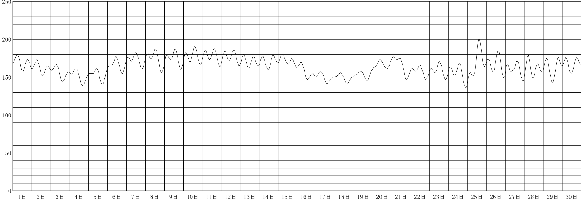
潮位 (cm) 1999年 9月
