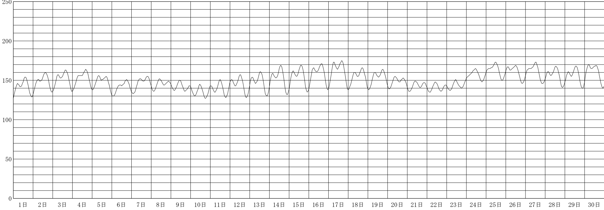
潮位 (cm) 1999年 6月
