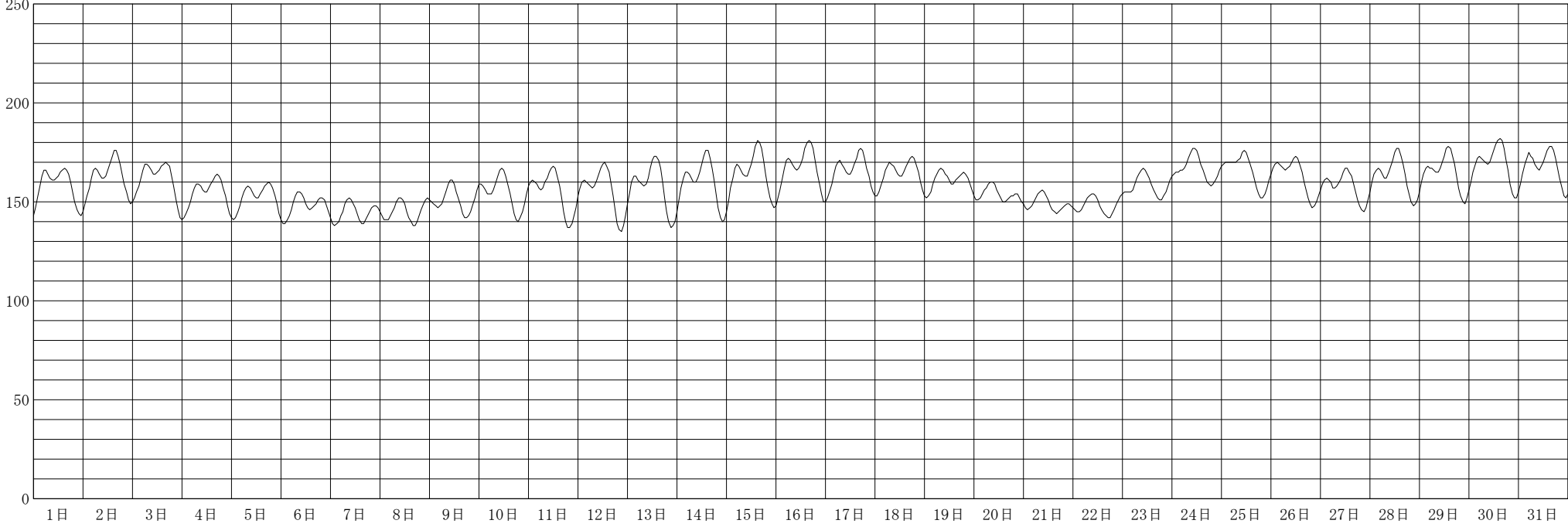
潮位 (cm) 1999年 7月
