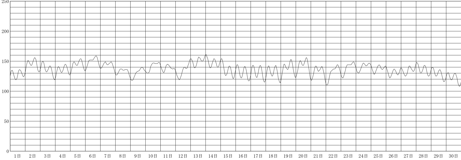
潮位 (cm) 1999年 4月
